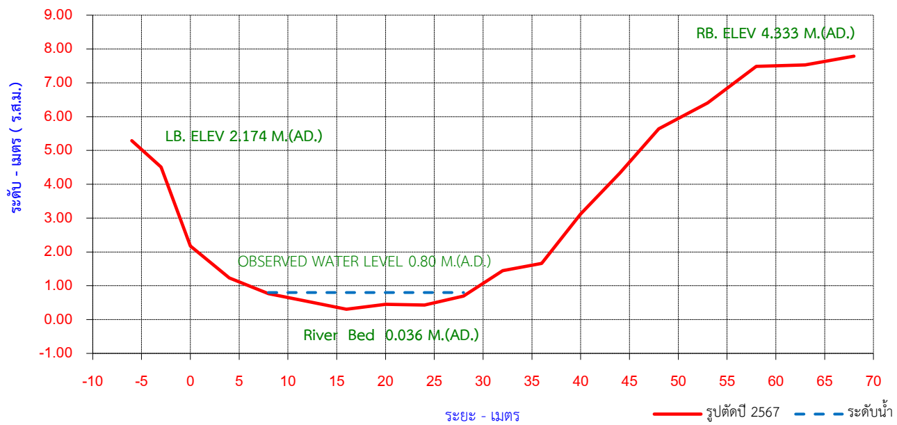
รูปตัดขวางลำน้ำ ปีน้ำ 2567 สถานี N.82 ห้วยน้ำรี อ.ท่าปลา จ.อุตรดิตถ์
